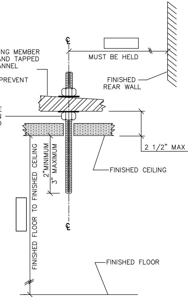
SECTION A-A
